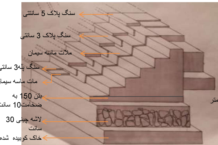
پله محوطه سازی با سنگ پلاک
