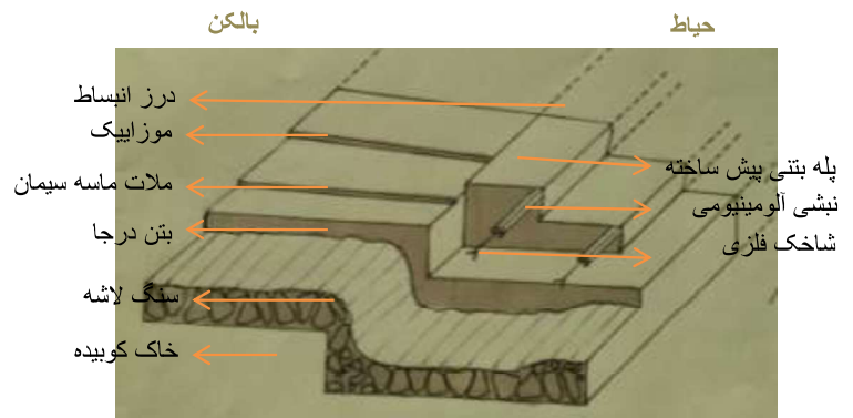
جزئیات پله بتنی پیش ساخته بین بالکن و حیاط
