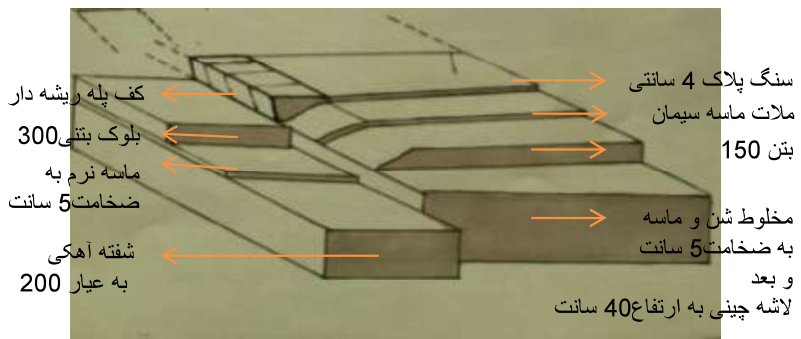
پله درب ورودی
