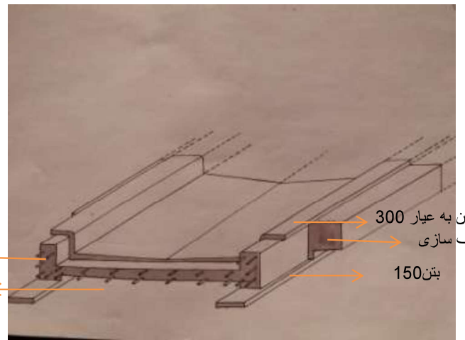
مقطع عرضی آبنا یا حوض
