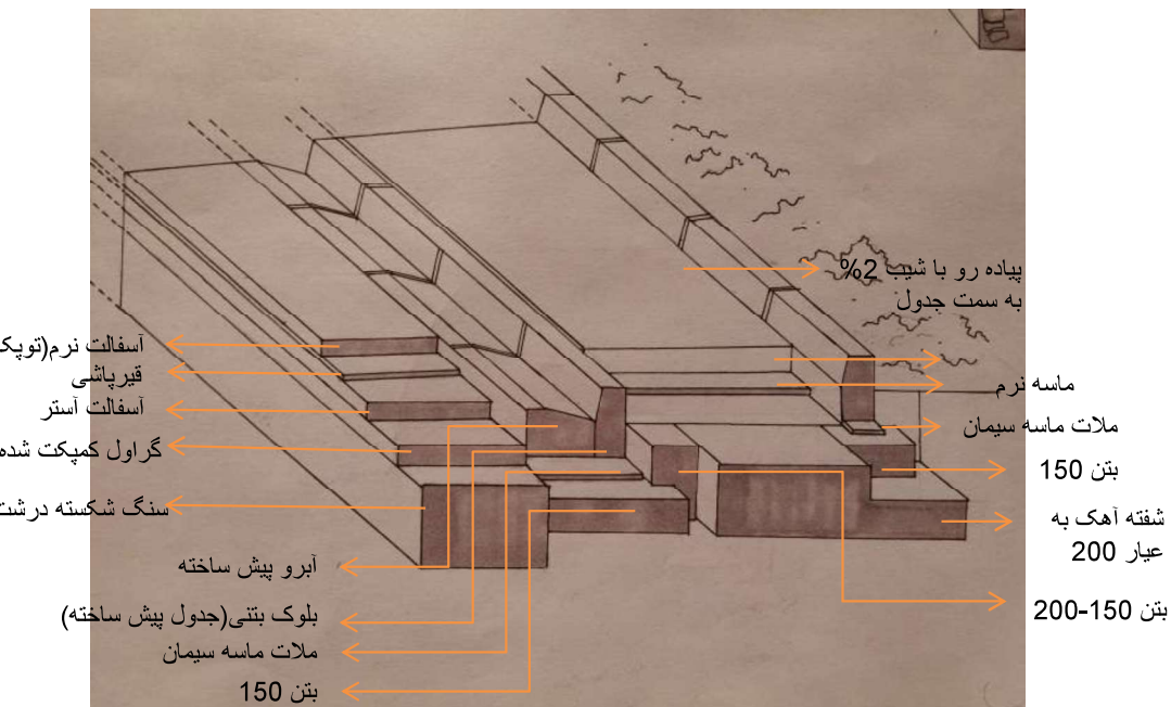
مقطع عرضی پیاده رو و جدول و آبروی کنار خیابان
