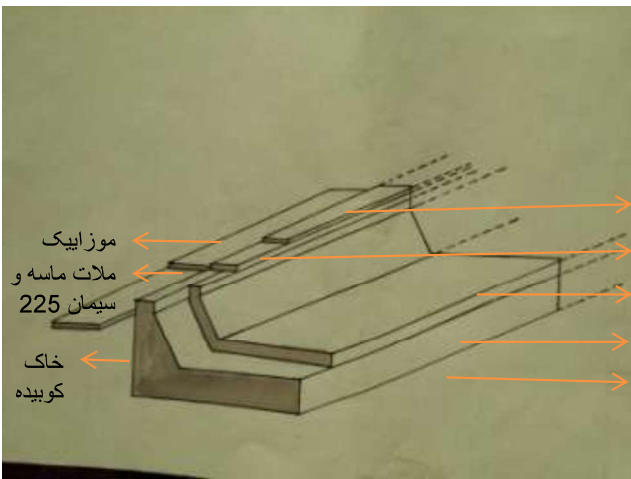
دیوار استخر
